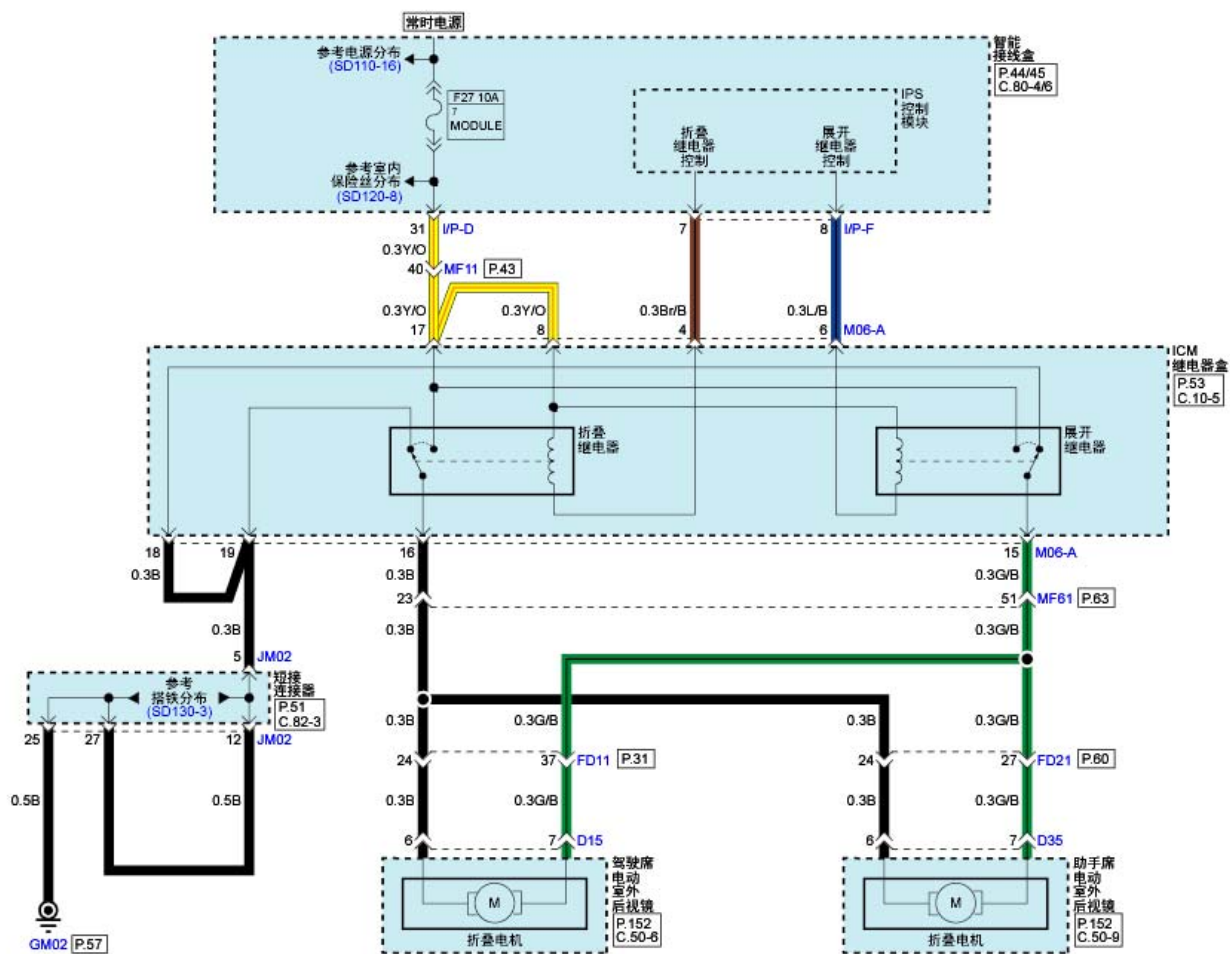
室外后视镜折叠系统(2)
